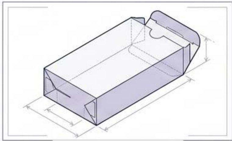
差し込み式折りたたみ箱（標準小売向け）
